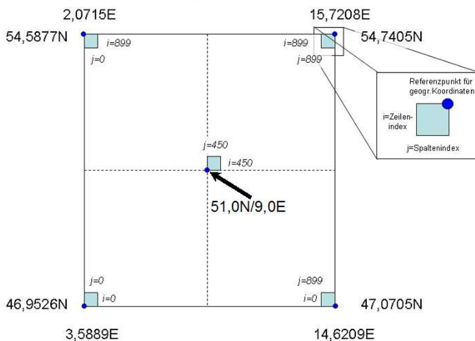
Abbildung 1: 1 x 1 km-Raster des nationalen Komposits (RADOLAN-Raster)
